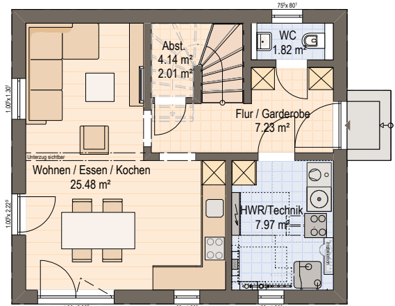
GRUNDRISS ERDGESCHOSS
