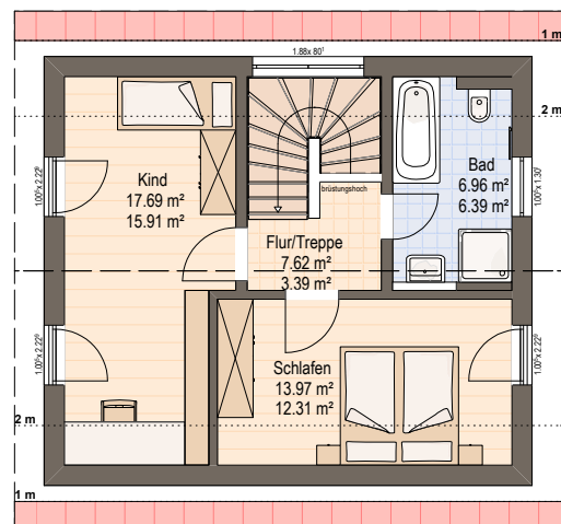
GRUNDRISS OBERGESCHOSS
