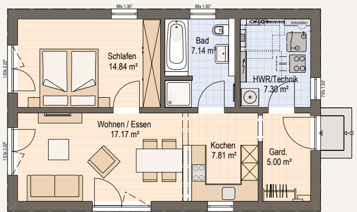
IHR GRUNDRISS
